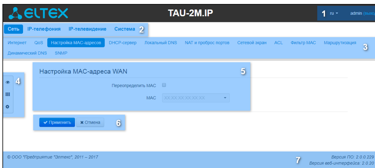
Рисунок 7 – Элементы навигации Web-конфигуратора
